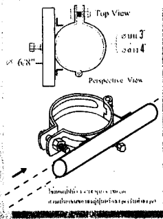
อุปกรณ์ประกอบการติดตั้ง AC-09
