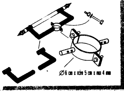
อุปกรณ์ประกอบการติดตั้ง CTT-48
