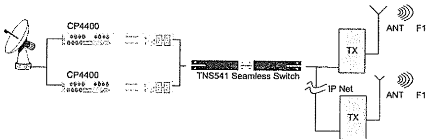
ภาพที่ 8 แนวทางการทดสอบ แบบที่ 1
