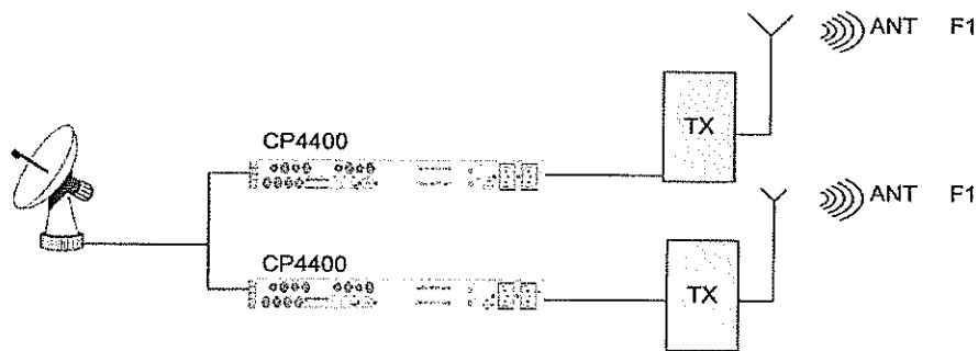
ภาพที่ 9 แนวทางการทดสอบ แบบที่ 2
