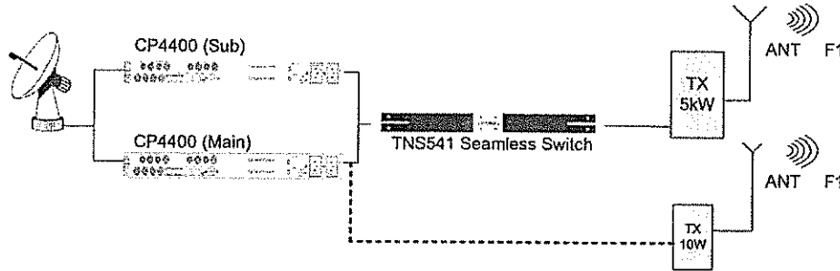
ภาพที่ 13 การต่ออุปกรณ์ใช้งานขณะทดสอบบนอาคารใบหยก
