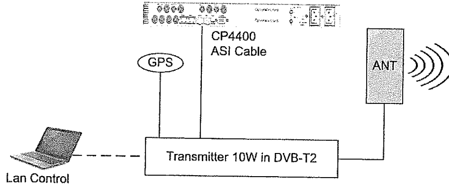
ภาพที่ 4 ลักษณะการต่ออุปกรณ์ในการทดลอง
