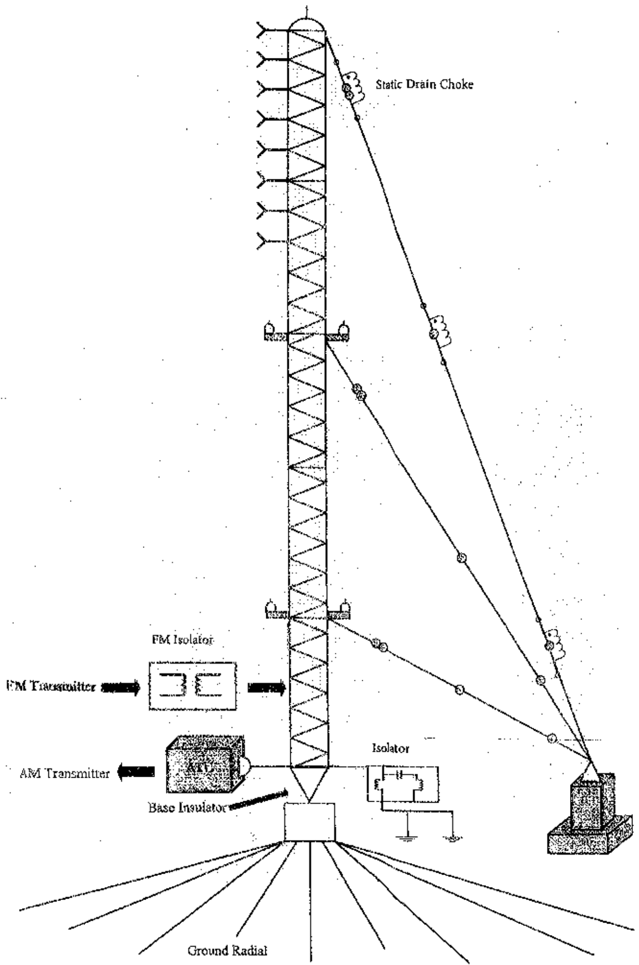
แนวทางการป้องกันไฟฟ้าสถิตย์ของสายอากาศ
