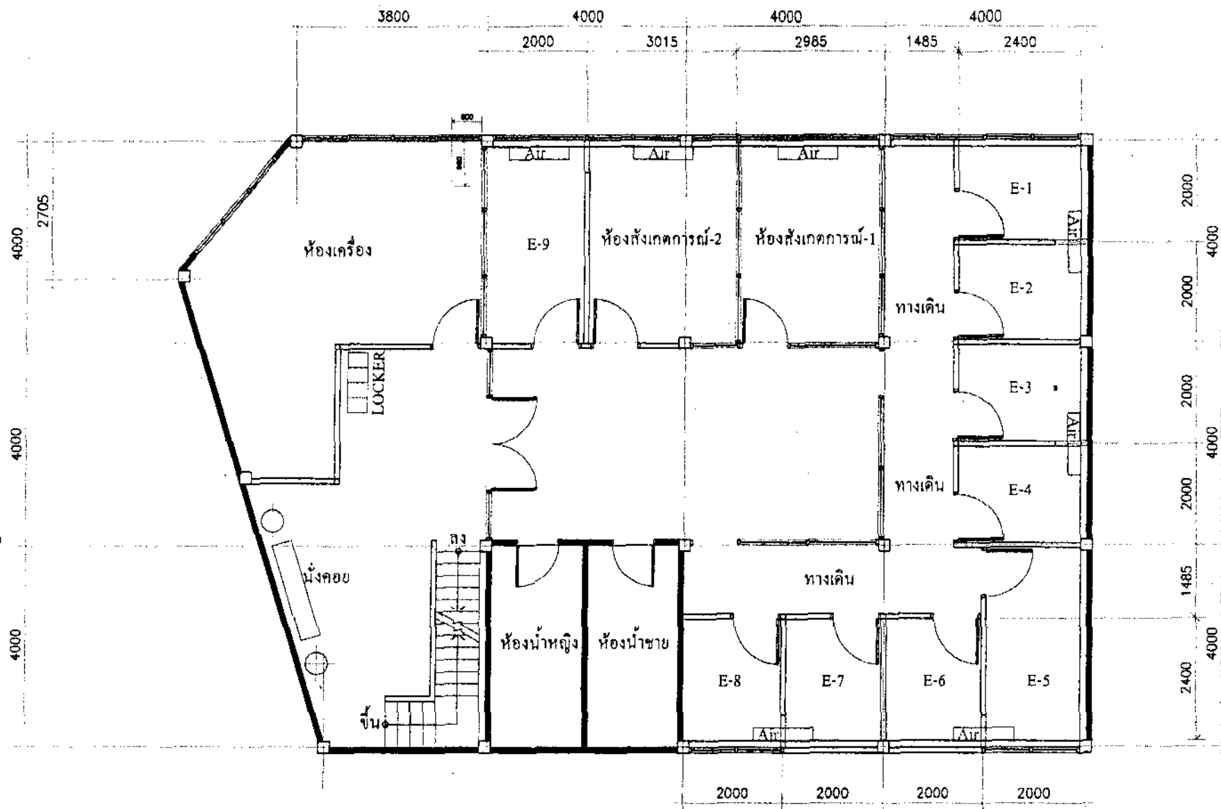
แบบแปลน ชั้น 2
